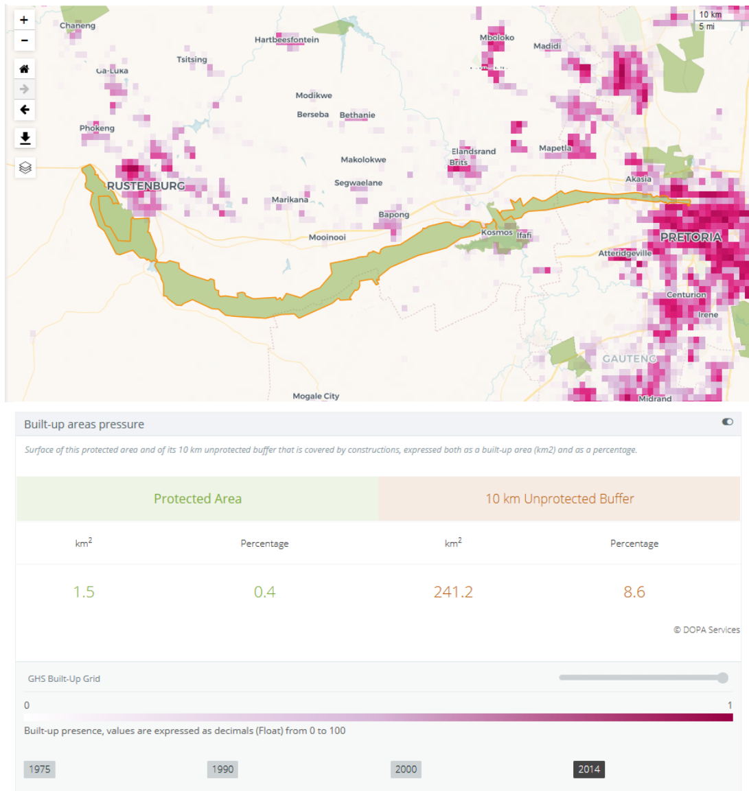
Gráfico 1. Mapa de la Reserva de la Biosfera de Magaliesberg (RSA) con las zonas urbanizadas actuales (arriba) y estimaciones cuantitativas de las zonas urbanizadas (en km 2 y %) para los años 1975, 1990, 2000 y 2014, indicadas en DOPA Explorer (parte inferior).
